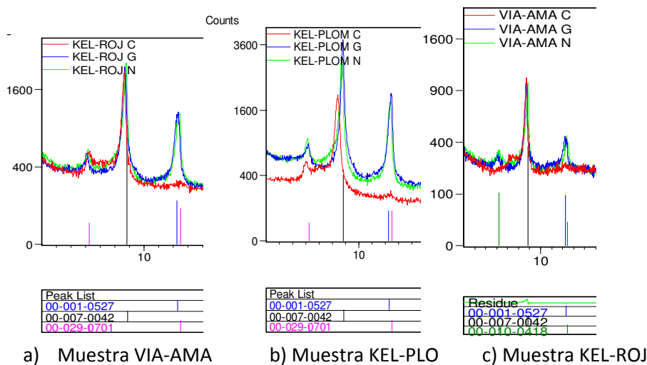
Figura N°5. Espectro de Difracción de Rayos – X e identificación de los minerales presentes de las muestras de Kellani.
