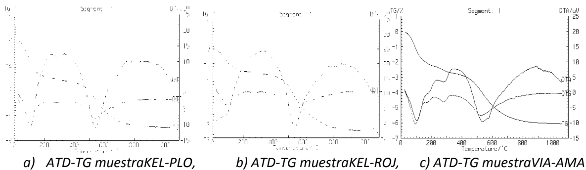
Figura N° 7. Termogramas de Análisis térmico diferencial y termo gravimetría a) muestra KEL-PLO, b) muestra KEL-ROJ, c) muestra VIA – AMA.
