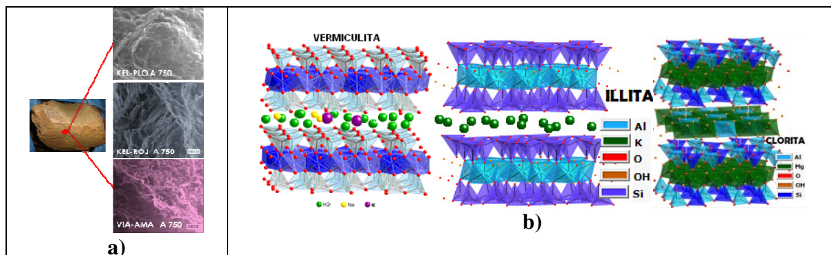
Figura N° 8. a) Microfotografías SEM que muestran la estructura laminar de los agregados en las muestras KEL-PLO, KEL-ROJ y VIA-AMA. b) estructuras laminares T-O-T y T-O-T-O de las arcilla que compones esas muestras
