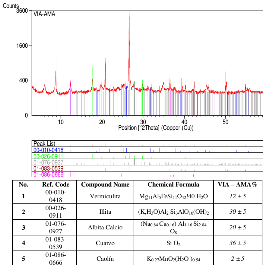
Figura N° 4. Espectro de Difracción de Rayos – X e identificación de los minerales presentes de las muestras de Viacha.
